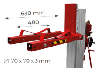
Support fûts et objets cylindriques
