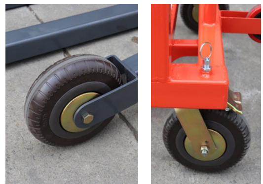
Roues caoutchouc dur (increvables) Ø 200 mm
